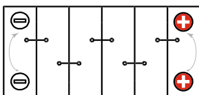
Schaltung Q
