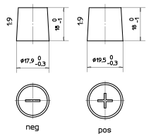
Anschlusspole 1
