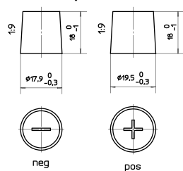
Anschlusspole 1
