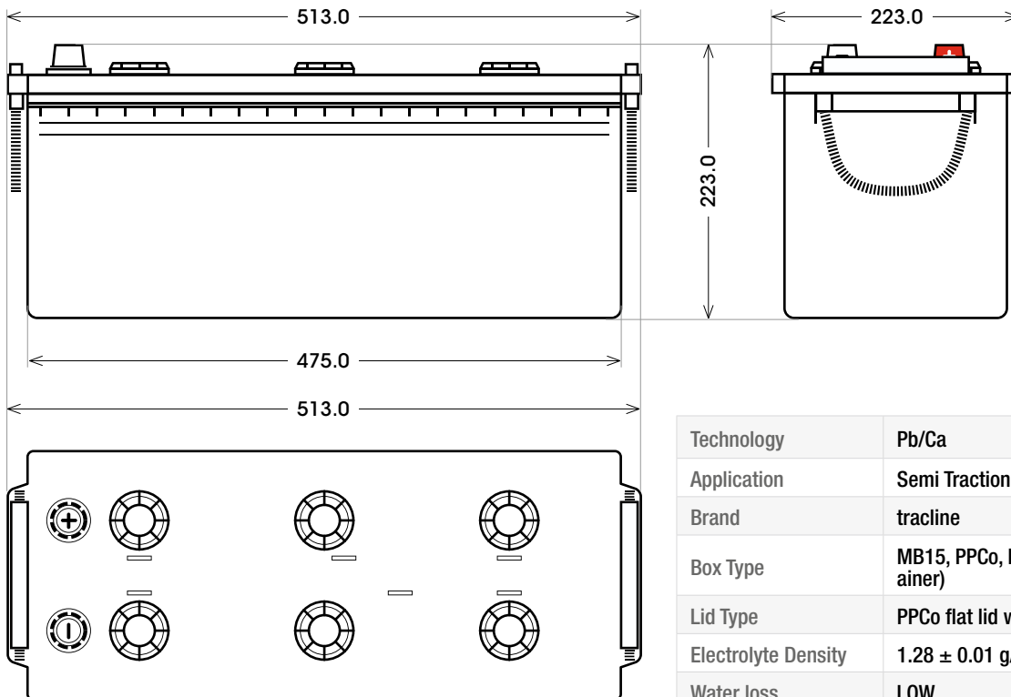
Bottom holder B00
