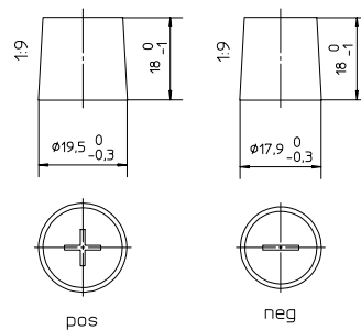
Anschlusspole 1
