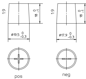
Anschlusspole 1
