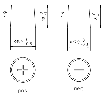
Anschlusspole 1
