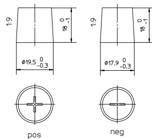
Anschlusspole 1
