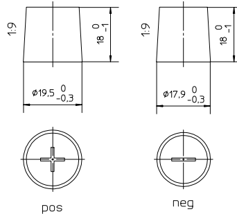
Anschlusspole 1
