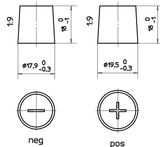
Anschlusspole 1
