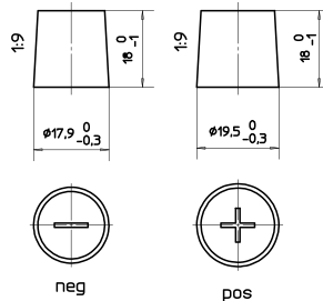
Anschlusspole 1
