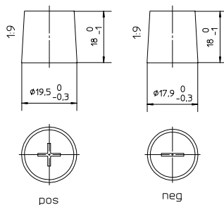
Anschlusspole 1
