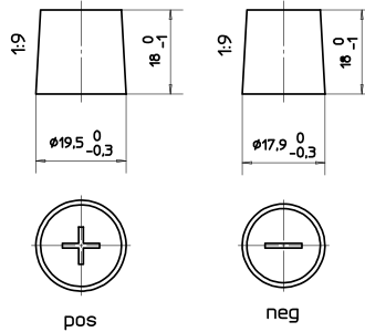
Anschlusspole 1
