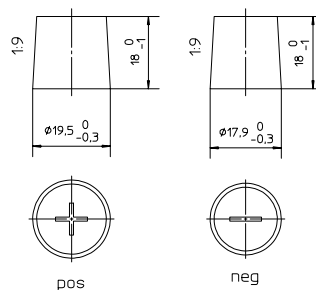
Anschlusspole 1
