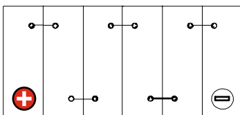
Schaltung 1
