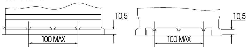
Bodenleiste B03
