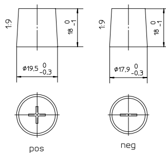
Anschlusspole 1
