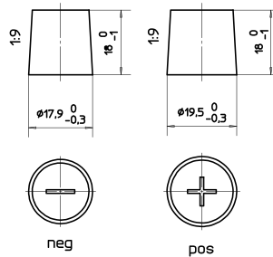
Anschlusspole 1
