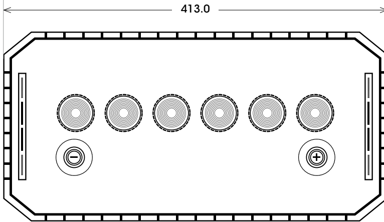
Bodenleiste B00
