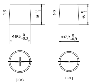
Anschlusspole 1
