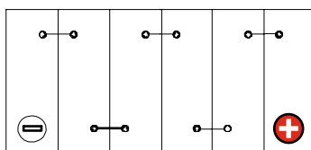
Schaltung 0
