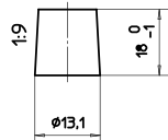
Anschlusspole 3
