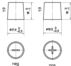
Anschlusspole 1
