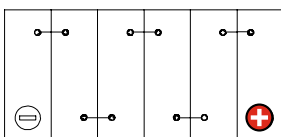
Schaltung 0
