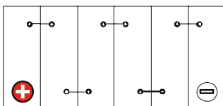
Schaltung 1
