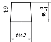
Anschlusspole 3
