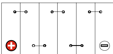
Schaltung 1
